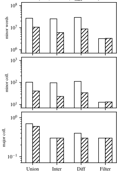
GC cost: stdlib vs par (1 domain) (IC1, n = 1M , b_{\max} = 128 )
