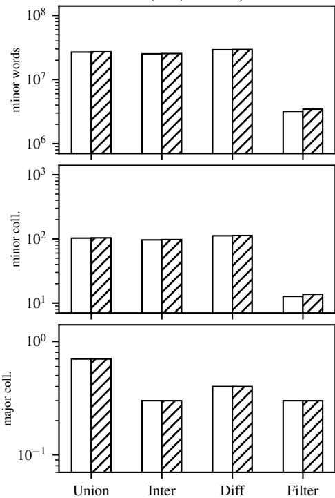
GC cost: stdlib seq vs par (1 domain) (IC1, n = 1M )
